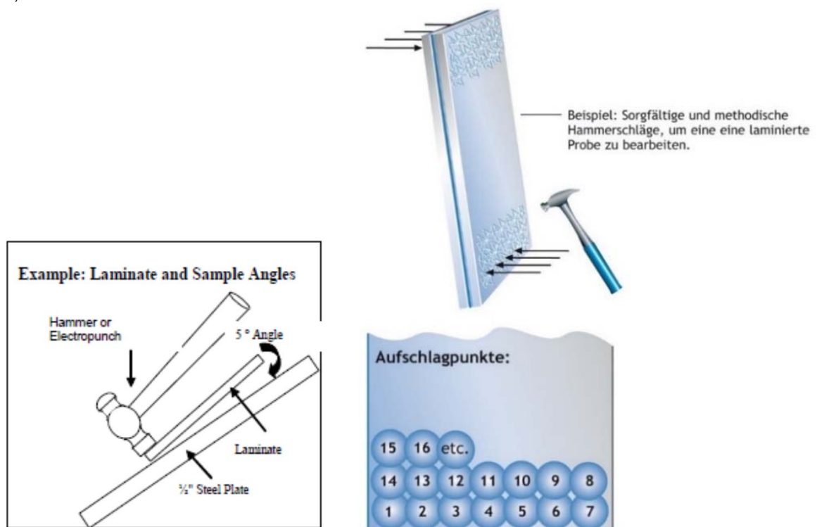
Abb. 3.1: Prüfdurchführung
